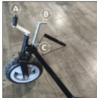
Frontleitrad (montiert)
