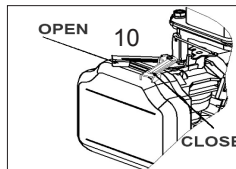
Chokehebel „CLOSE“
