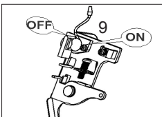
Zündschalter „ON“
