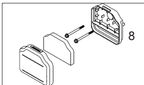
Luftfilter reinigen
