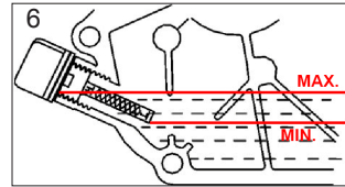
Ölstand
